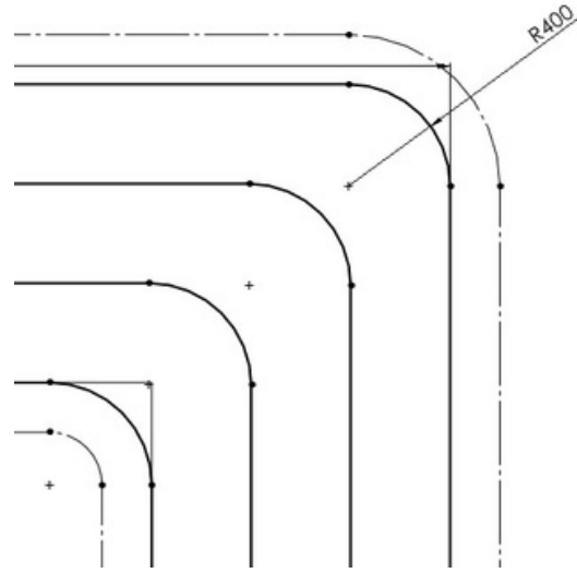
Şekil 7. 400 mmyarıçapında viraj
